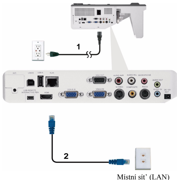
Místní síť (LAN)
